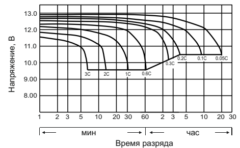
Разрядные характеристики
